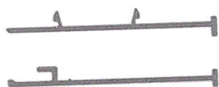
Figure 1.3 : Profil d'habillage du rail aluminium
