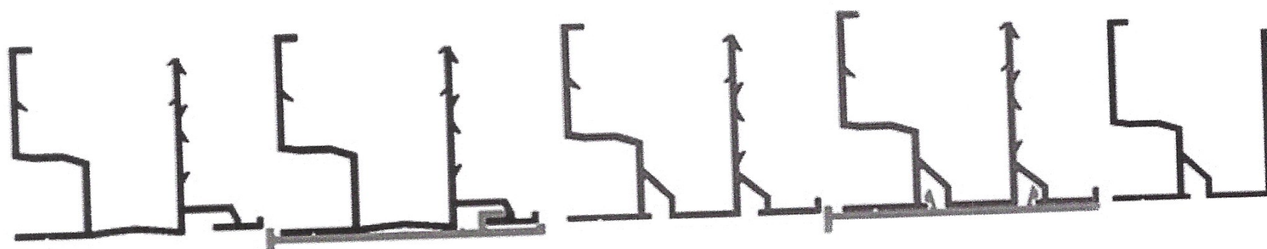
Figure 1.1 : Rails aluminium extérieurs sans et avec le cache rail
