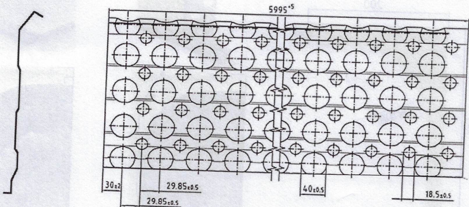
Figure 1.5 : Armature métallique plate
